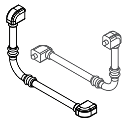
PIPE: G2 3mm dia. Length 40mm 90° Bend
